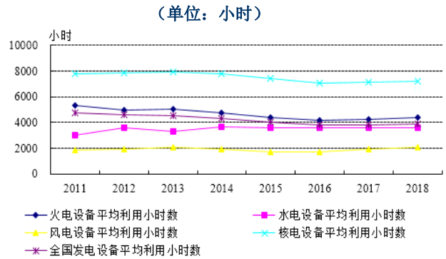
图 8：2011 年以来全国电力设备利用小时数情况
